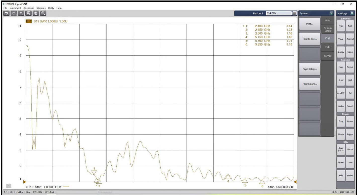
VSWR图
