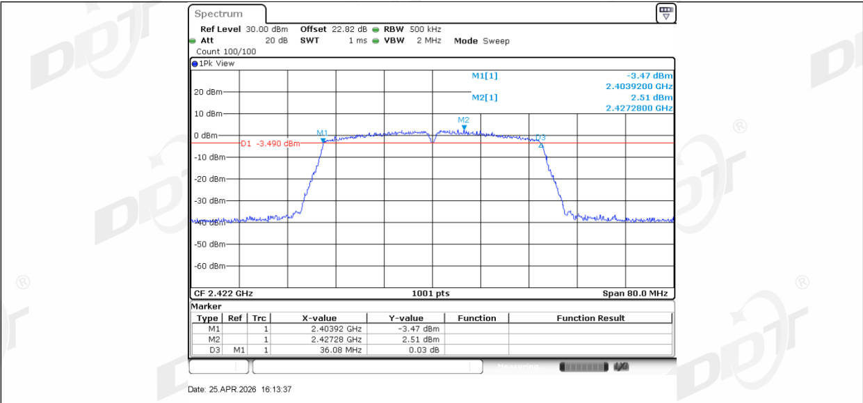
11N40MIMO_Ant2_2422
