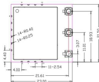
模组俯视图
