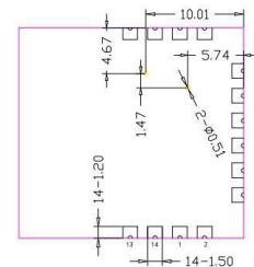
模组底视图
