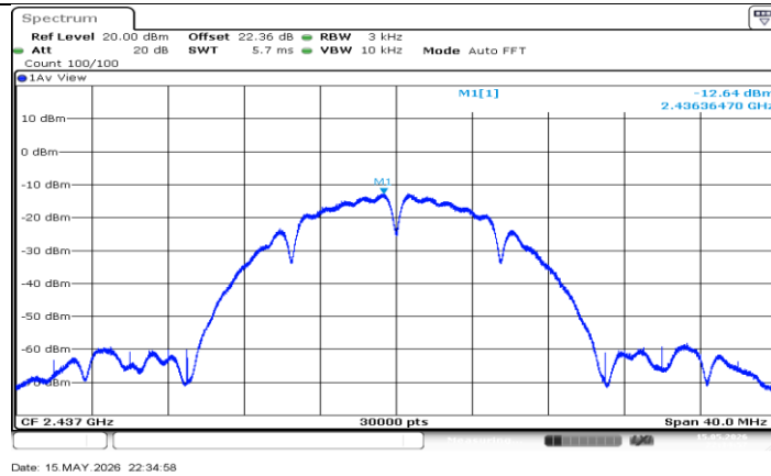
11B-CDD_Ant1_2437
