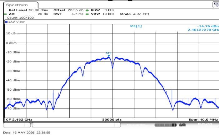
11B-CDD_Ant0_2462
