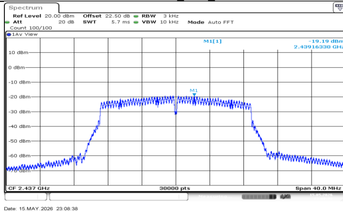
11N20MIMO_Ant0_2437
