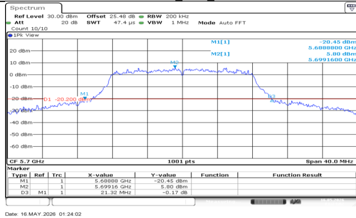
11A-CDD_Ant0_5700
