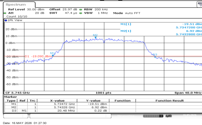
11A-CDD_Ant0_5745
