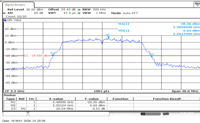
11A-CDD_Ant0_5500
