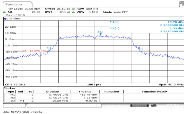
11A-CDD_Ant0_5720
