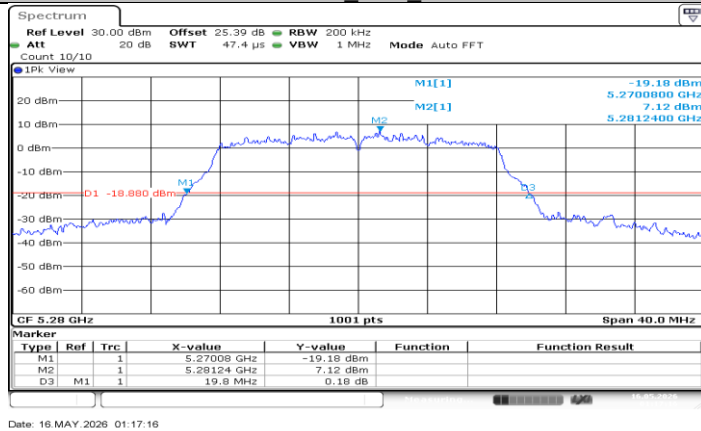
11A-CDD_Ant0_5280
