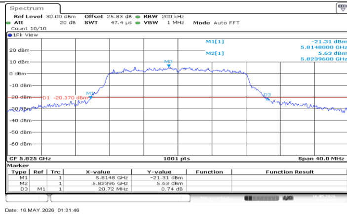
11A-CDD_Ant0_5825
