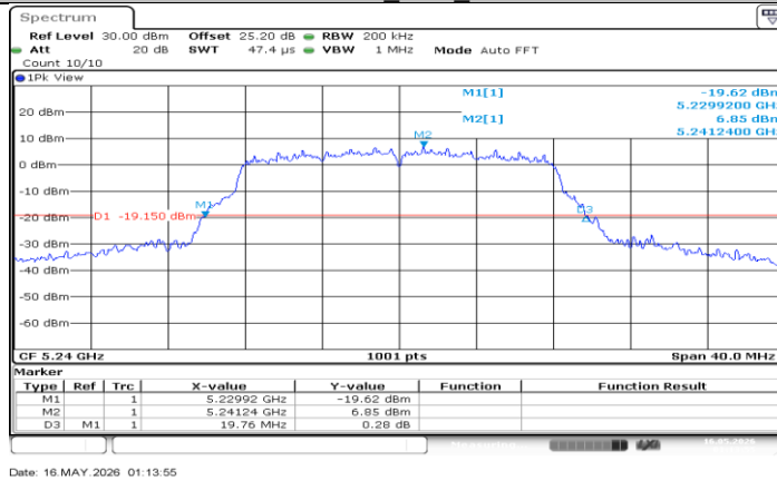
11A-CDD_Ant0_5240
