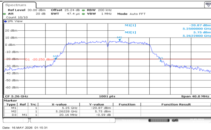
11A-CDD_Ant0_5260
