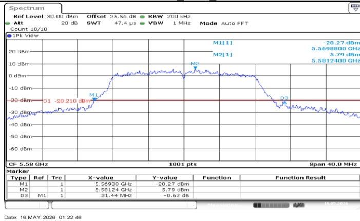
11A-CDD_Ant0_5580
