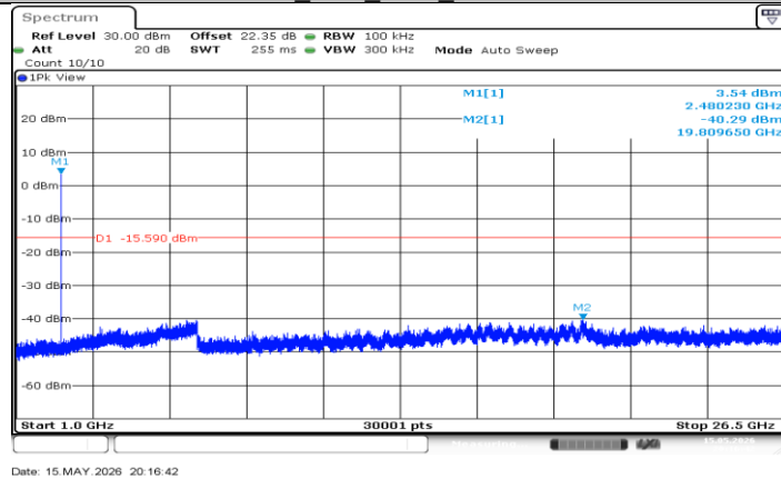
DH5_Ant2_2480_1000~26500
