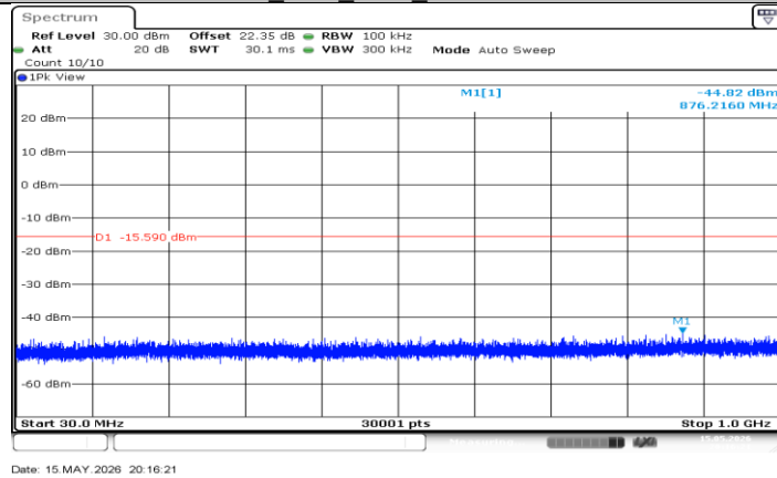
DH5_Ant2_2480_30~1000
