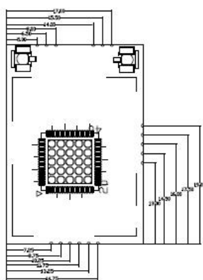
模组主视图
