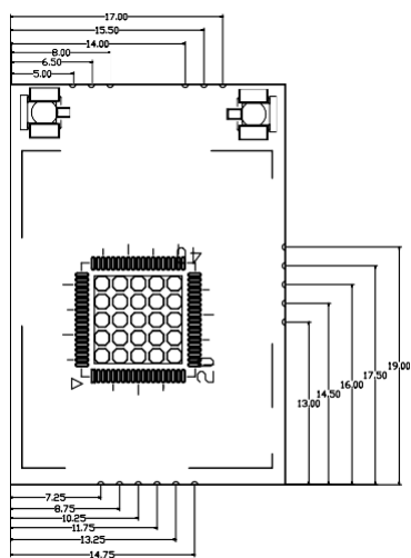
模组主视图
