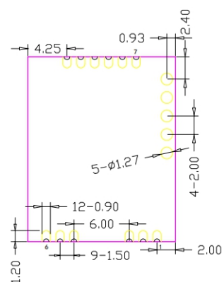
模组底视图
