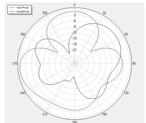
Theta=90 freq=2400MHz
