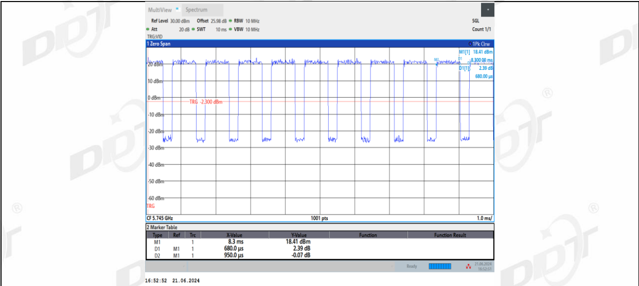
11AC20MIMO_Ant2_5745
