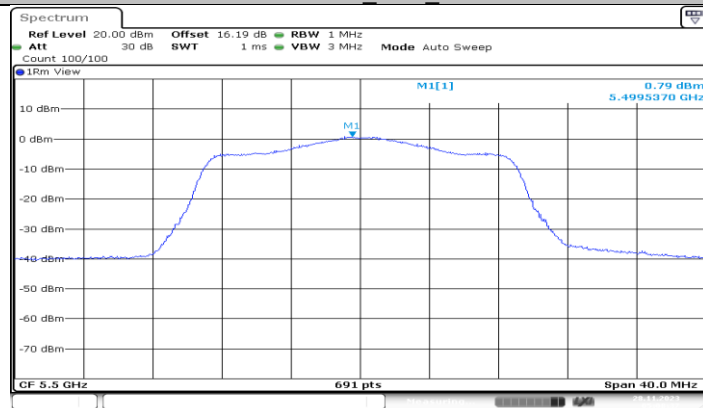
11N20MIMO_Ant1_5500
