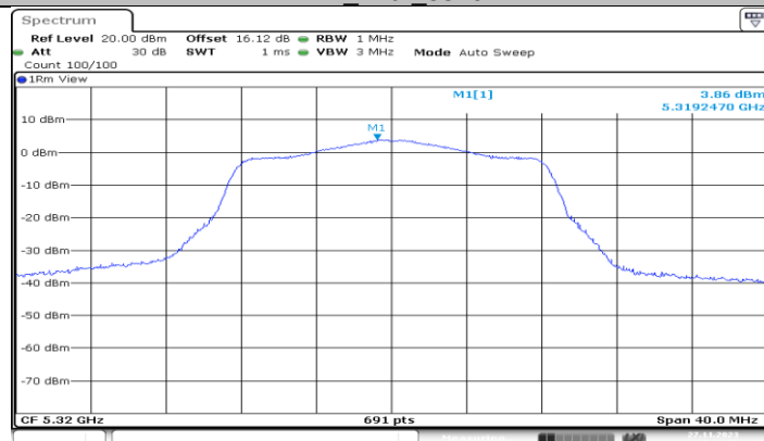
11A_Ant1_5320
