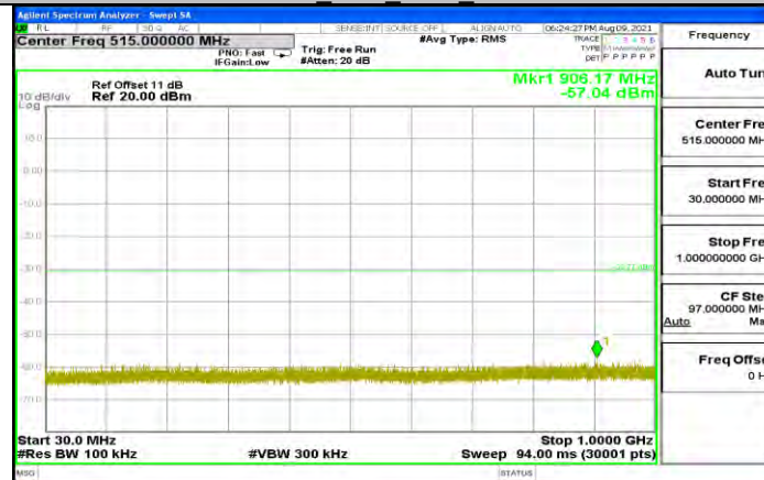
11N40MIMO_Ant2_2422_30~1000
