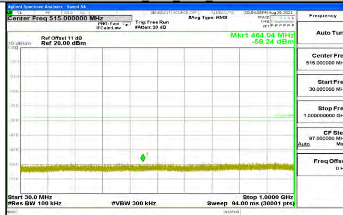
11N20MIMO_Ant2_2437_30~1000
