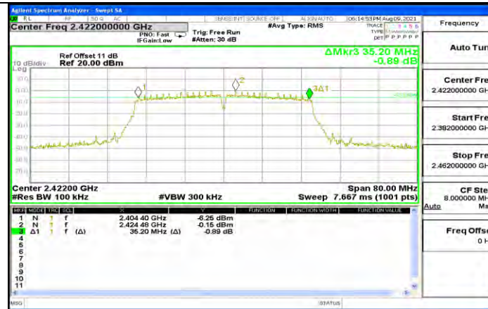
11N40MIMO Ant1 2422
