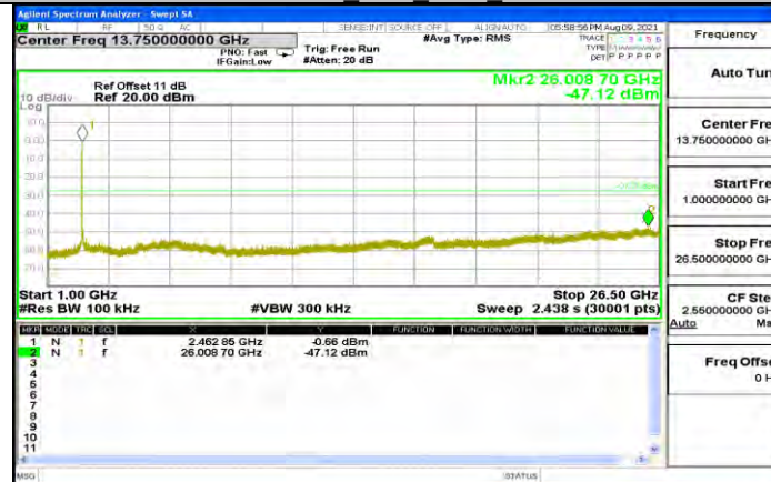
11N20MIMO_Ant1_2462_1000~26500
