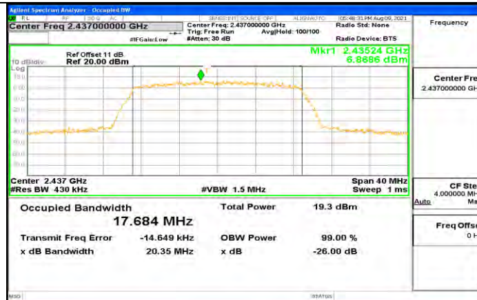
11N20MIMO Ant2 2437
