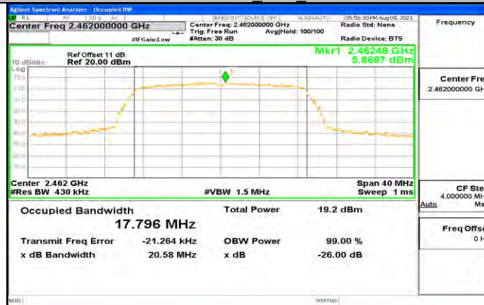
11N20MIMO Ant1 2462
