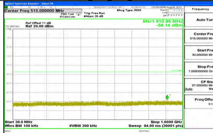
11N20MIMO_Ant1_2462_30~1000
