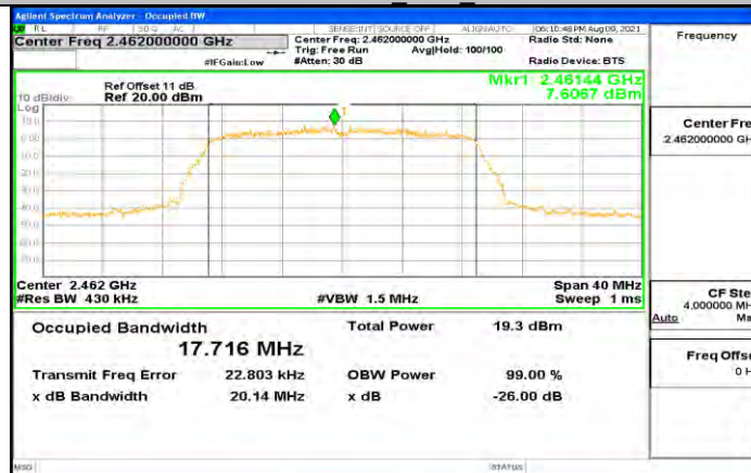
11N20MIMO Ant2 2462
