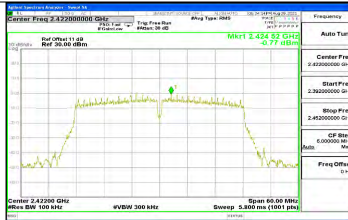
11N40MIMO_Ant2_2422_0~Reference
