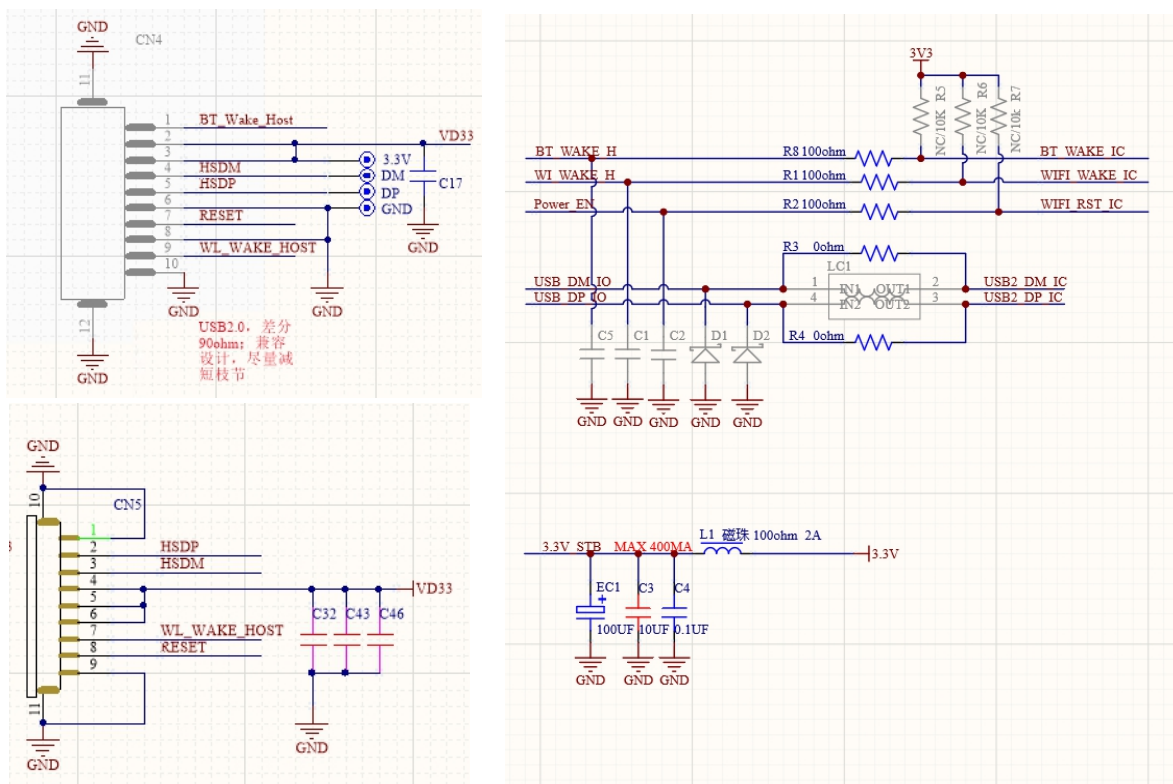
圖 10-1 參考原理圖
