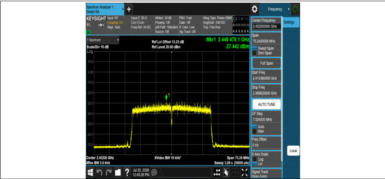
11AX40MIMO_Ant2_2452
