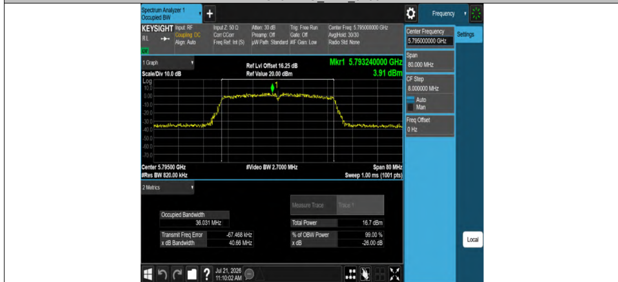
11AC40MIMO_Ant2_5795
