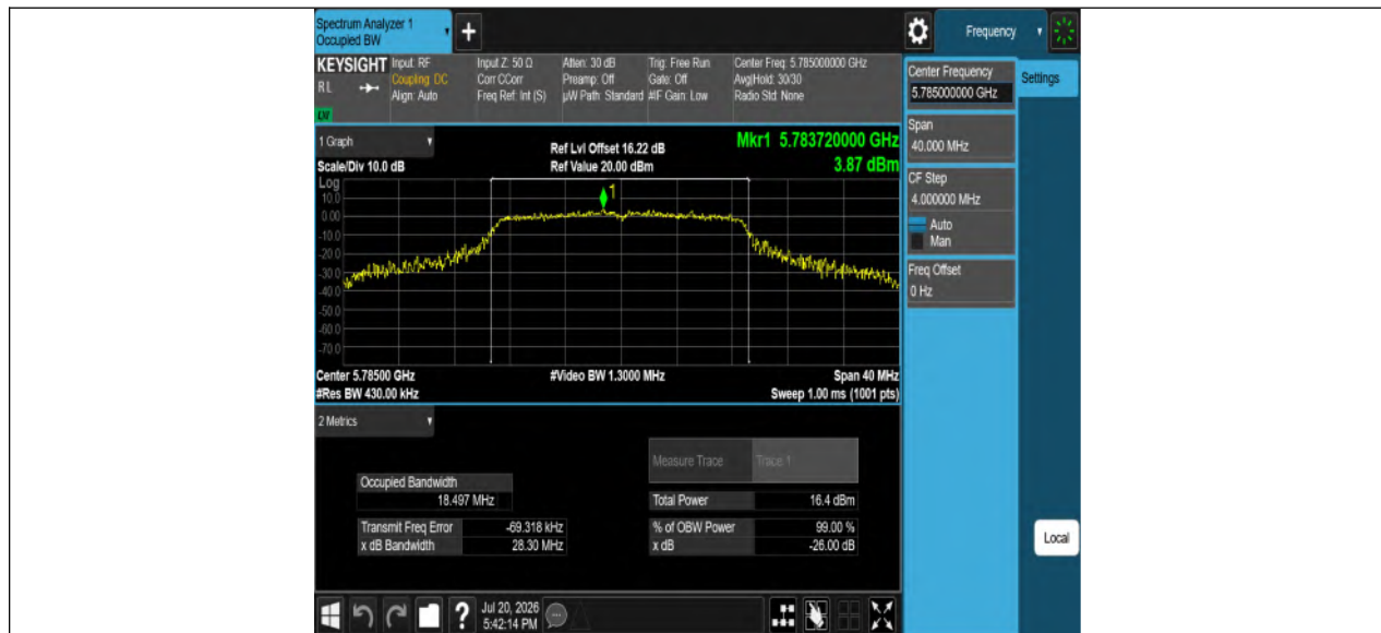
11N20MIMO_Ant2_5785
