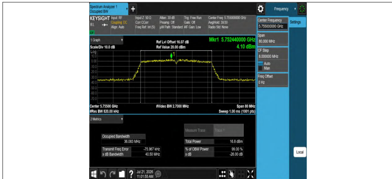
11AC40MIMO_Ant2_5755
