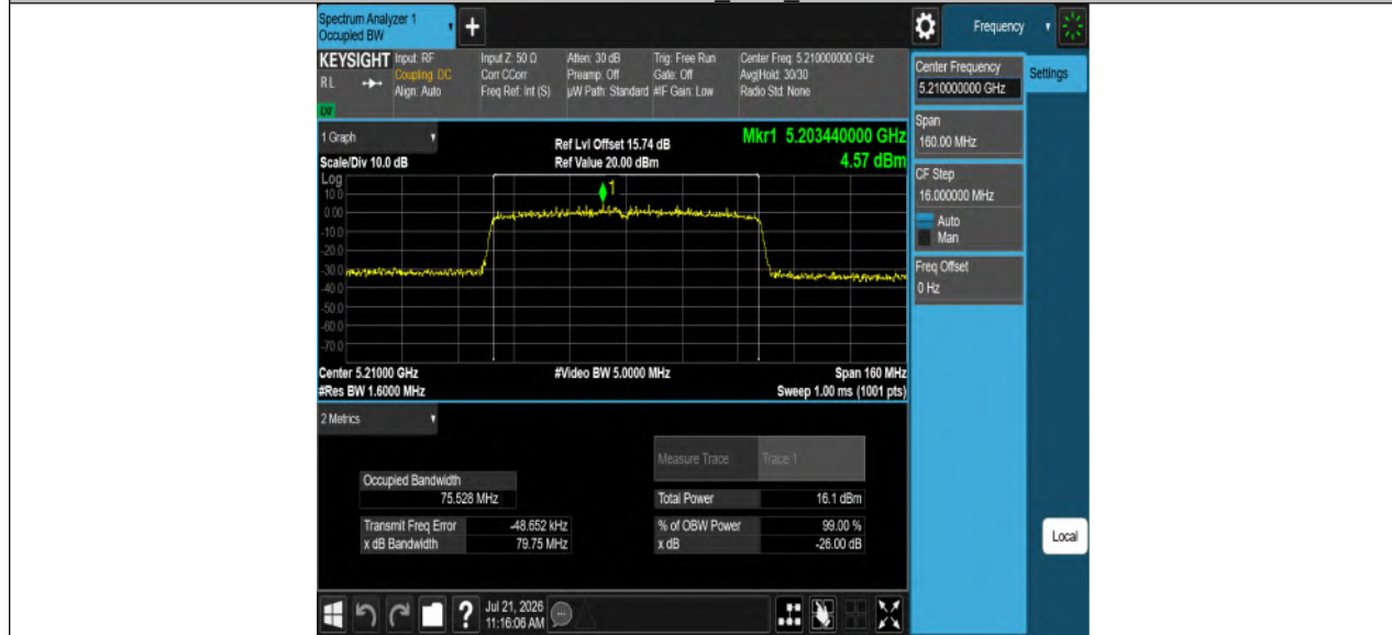
11AC80MIMO_Ant2_5210
