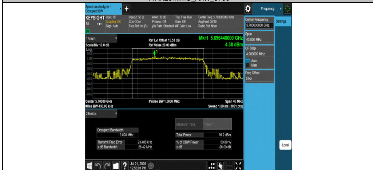
11AX20MIMO_Ant2_5700
