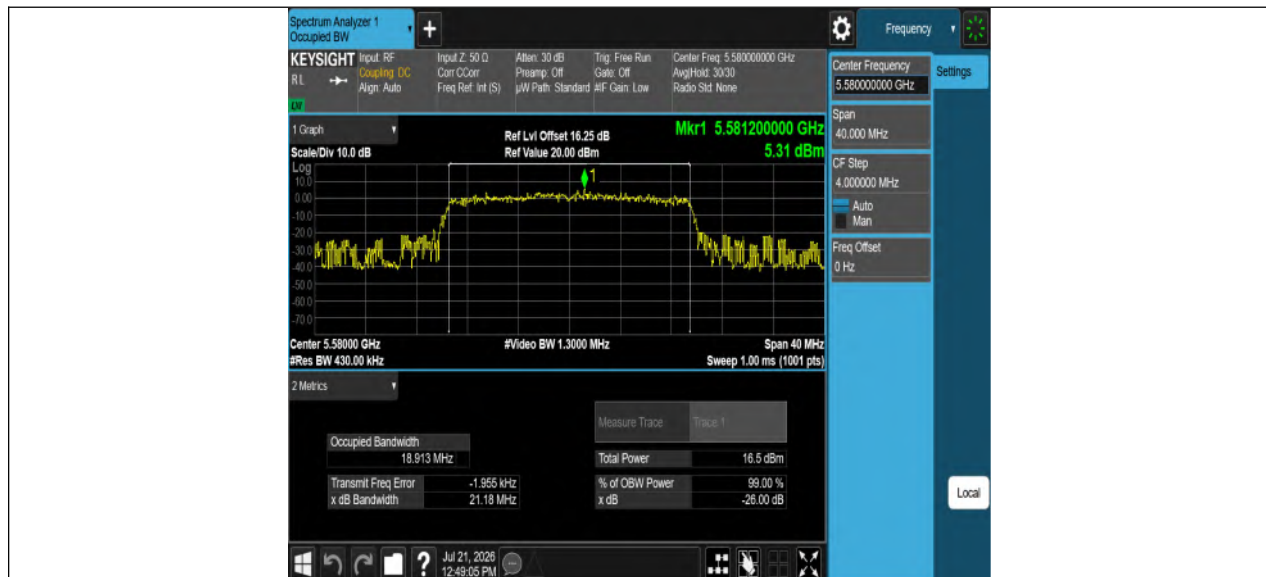
11AX20MIMO_Ant2_5580
