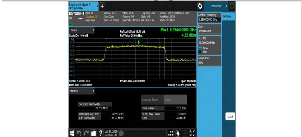
11AX80MIMO_Ant2_5290
