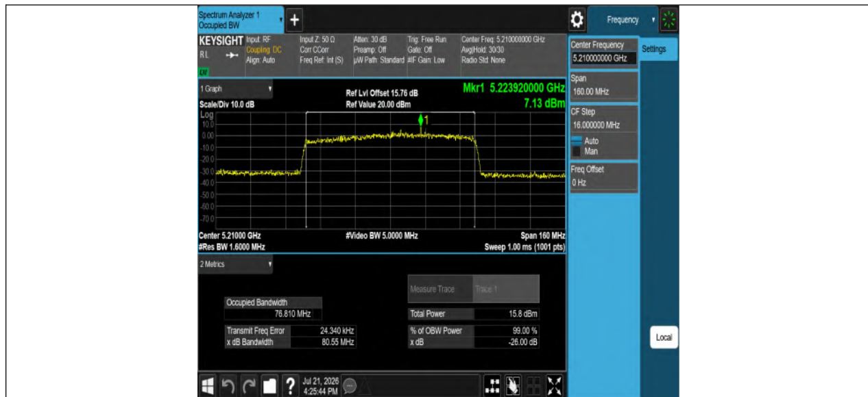
11AX80MIMO_Ant1_5290
