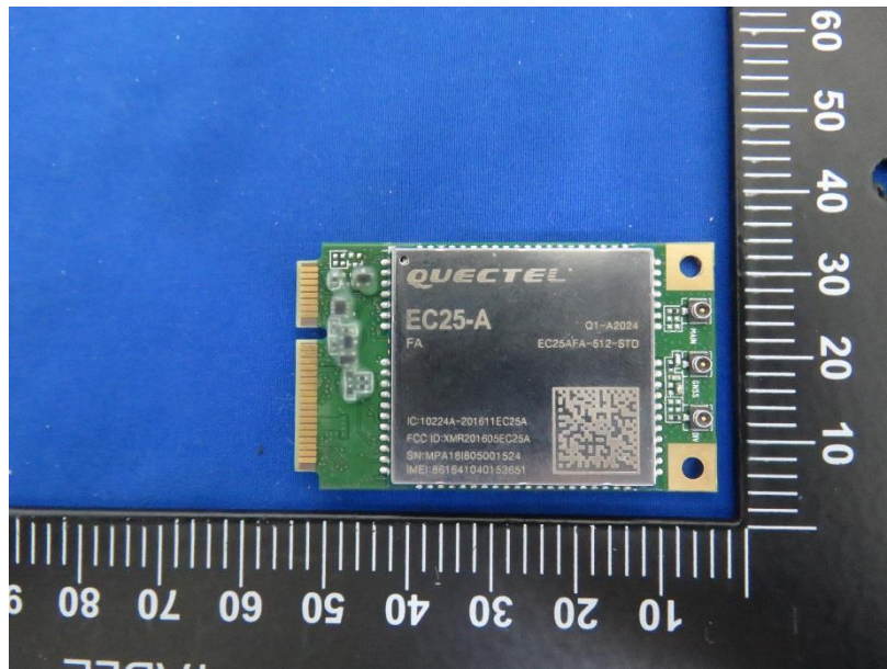
LTE Module
