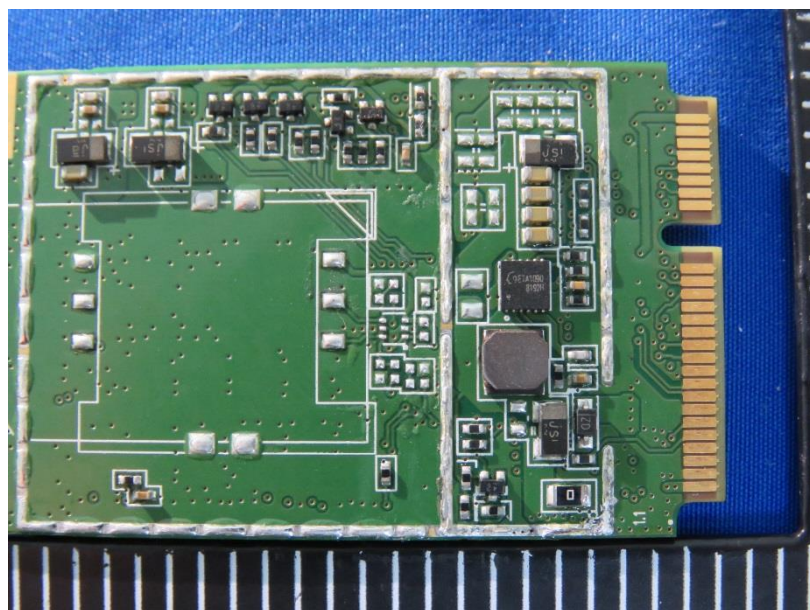
LTE Module
