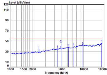
BLE_1M_TX_CH_20_Horizontal-Avg
