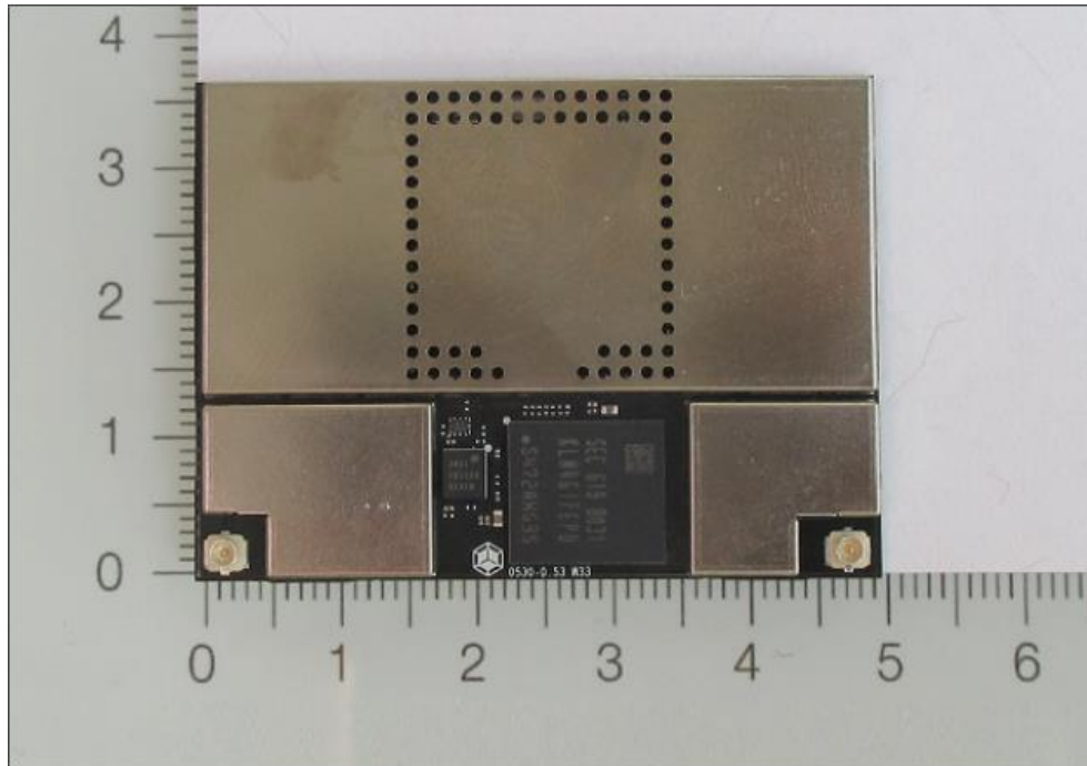
(2) EUT Photo
