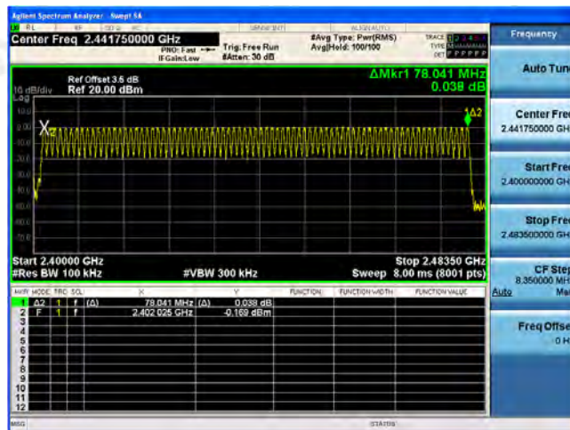
GFSK
