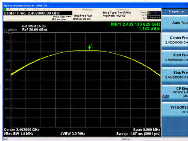
CH00
