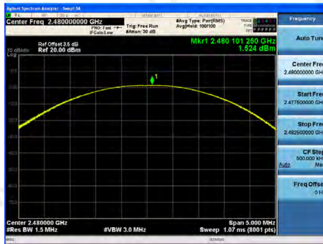
CH78
