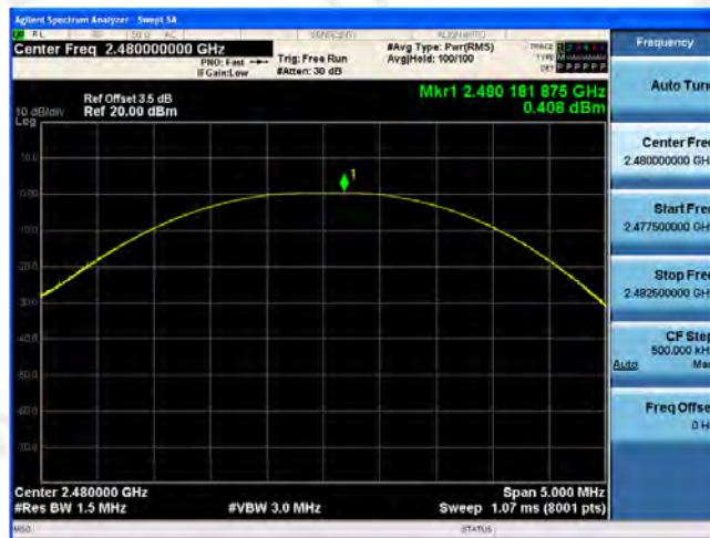
CH78
