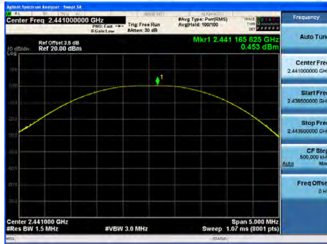
CH39
