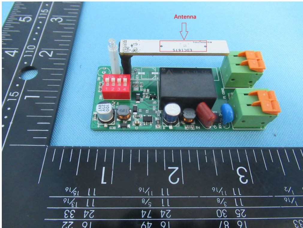
(3) EUT Photo
