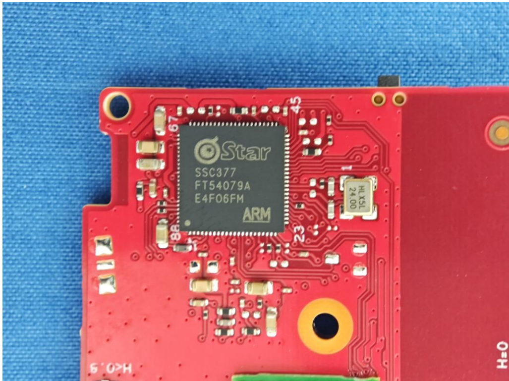
12) EUT Photo
