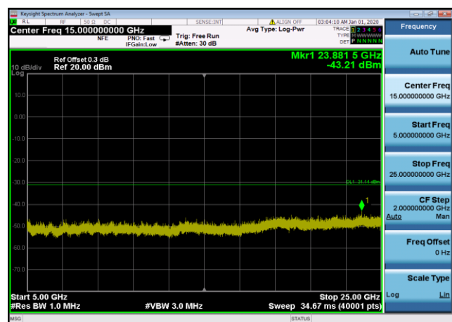
2480MHz,Plot 5,5000MHz~25000MHz
