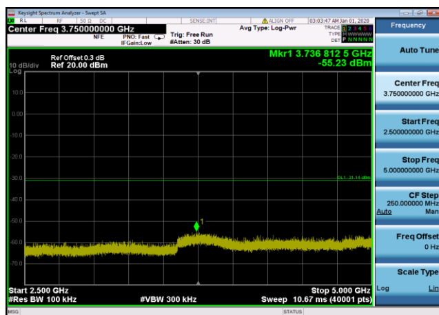
2480MHz,Plot 4,2500MHz~5000MHz
