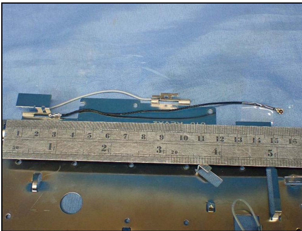
Antenna: BLE_baseline
