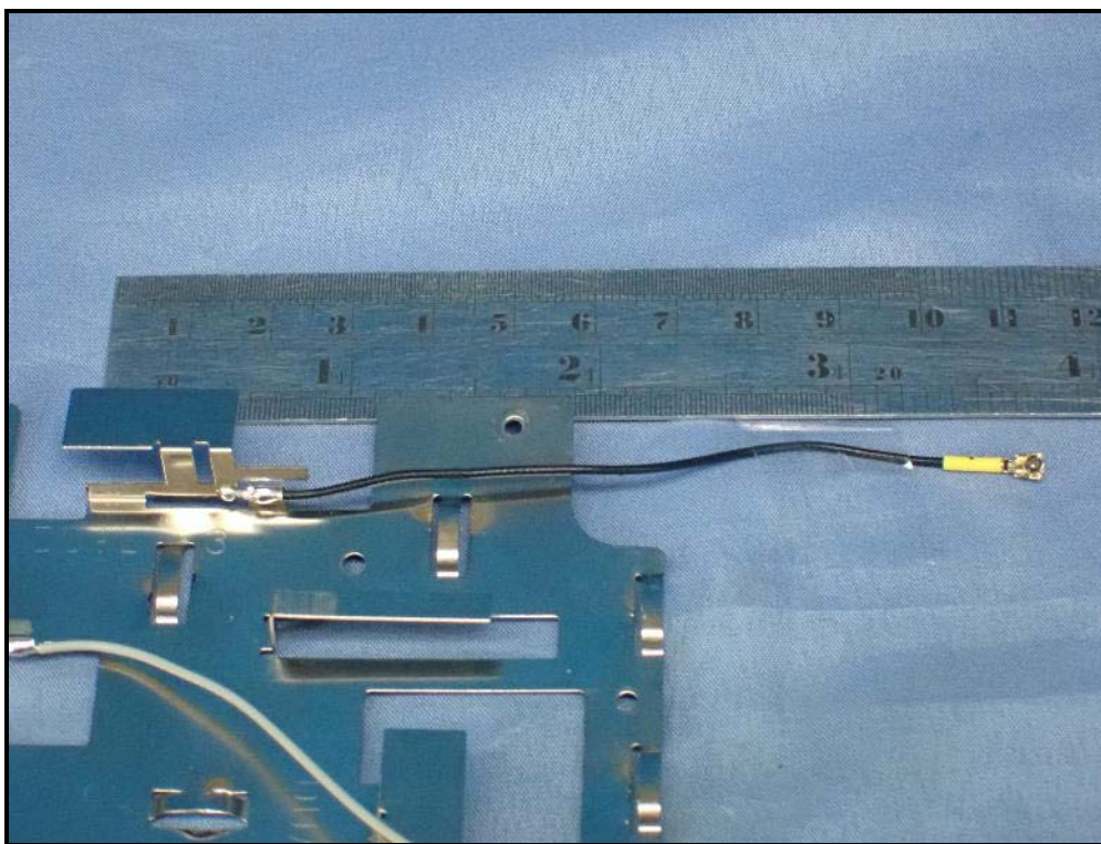
Antenna: DUAL3
