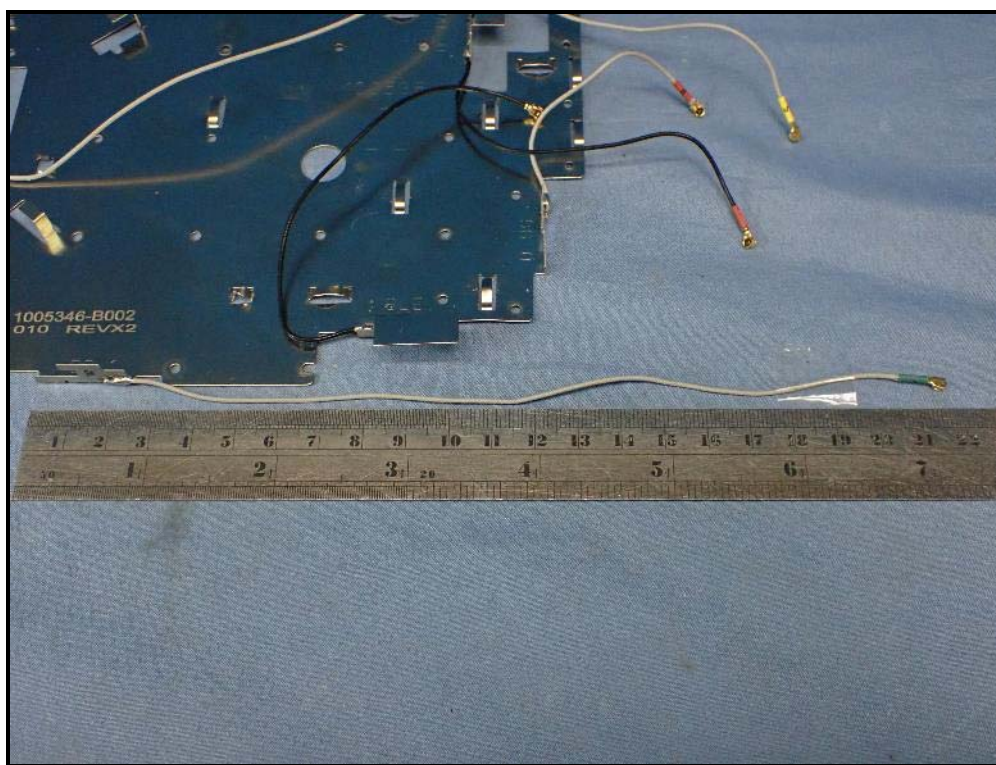
Antenna: 5G1_baseline
