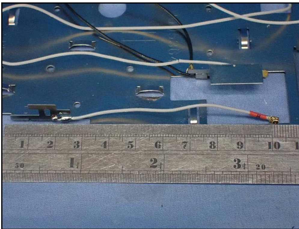
Antenna: 5G0_baseline
