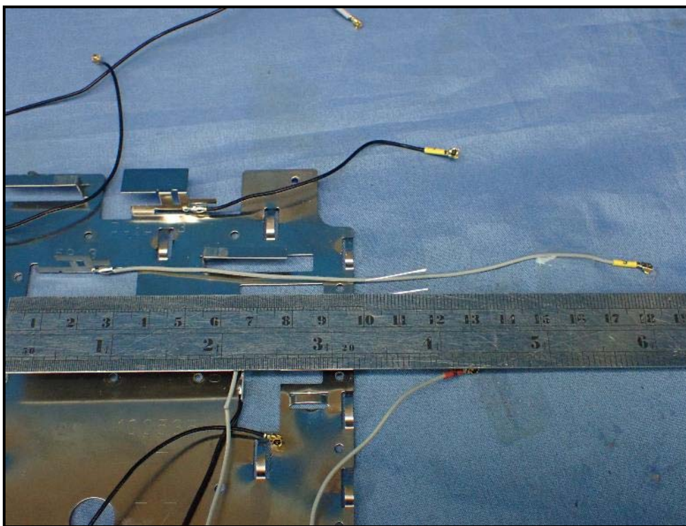
Antenna: 5G3_baseline
