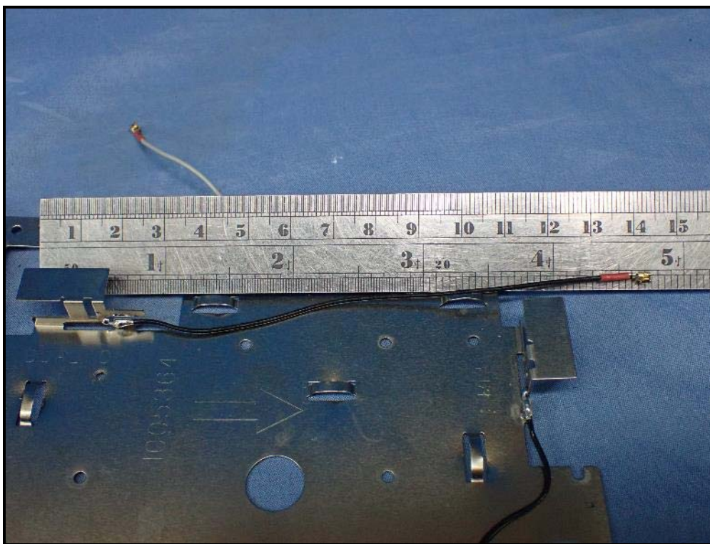
Antenna: DUAL0
