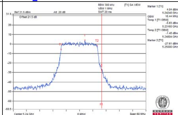
802.11a_Chain 7 / CH48
