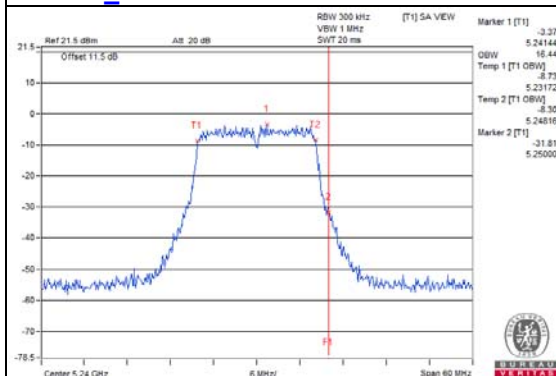
802.11a_Chain 4 / CH48
