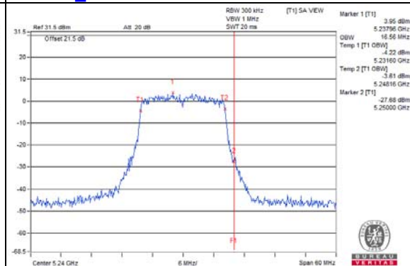
802.11a_Chain 5 / CH48
