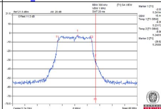
802.11a_Chain 3 / CH48
