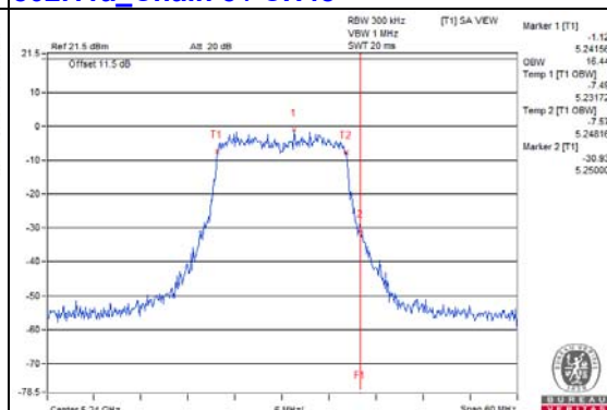
802.11a_Chain 7 / CH48
