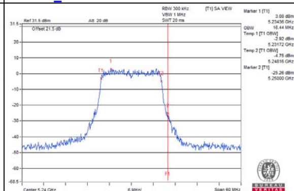
802.11a_Chain 3 / CH48
