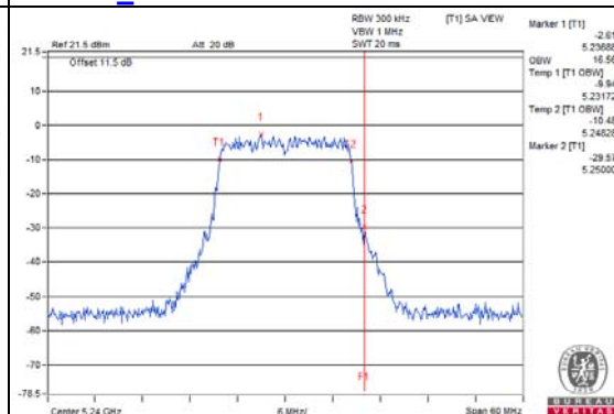
802.11a_Chain 5 / CH48
