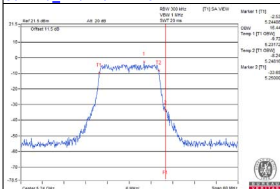
802.11a_Chain 6 / CH48
