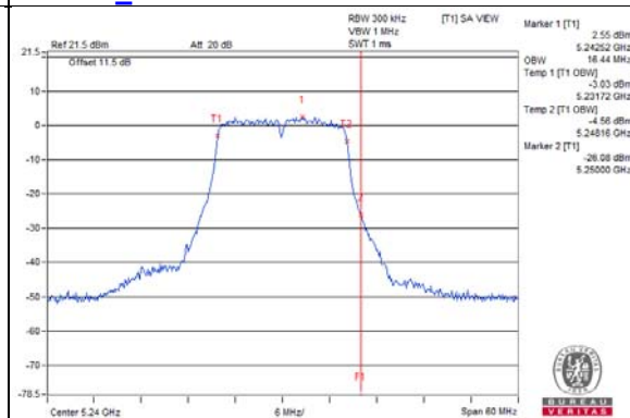
802.11a_Chain 3 / CH48
