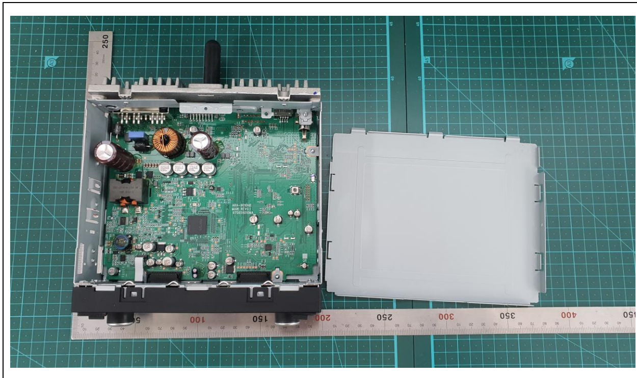
ARA-9010H Inside
