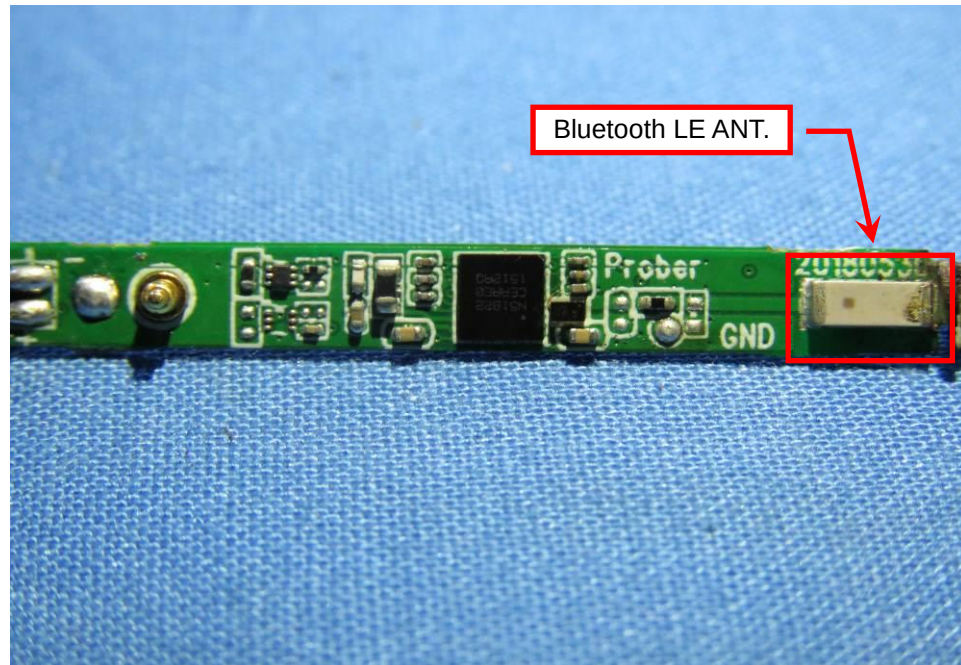
EUT Photo (6)
