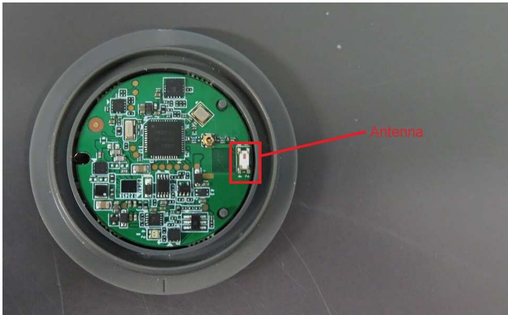
Antenna
