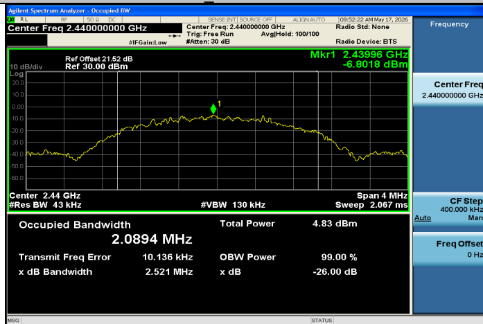
BLE 2M-Ant1-2440
