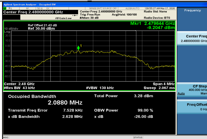
BLE 2M-Ant1-2480
