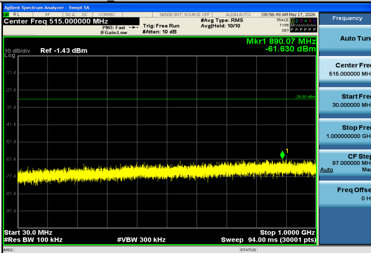
BLE_2M-Ant1-2480-30~1000-PASS
