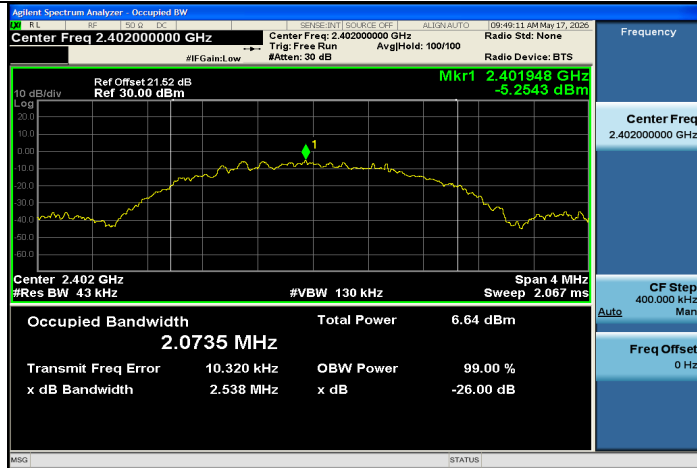
BLE 2M-Ant1-2402
