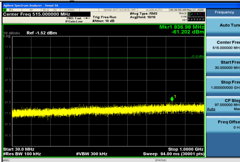
BLE 1M-Ant1-2402-30~1000-PASS
