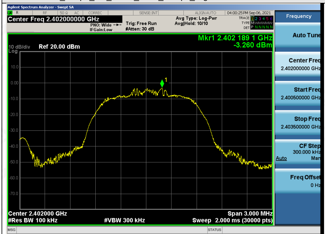
Test_Graph_EDR_ANT1_2402_2Mbps_Reference Level
