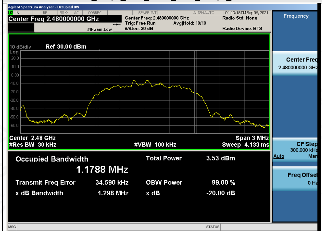
Test_Graph_EDR_ANT1_2480_3Mbps_OBW
