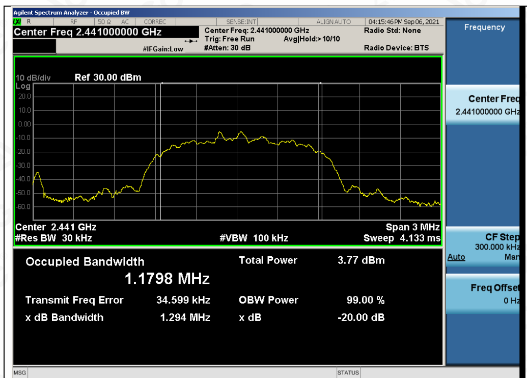
Test_Graph_EDR_ANT1_2441_3Mbps_OBW
