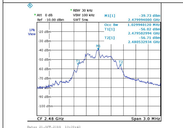
Figure 31. 2480.0 MHz, BLE
