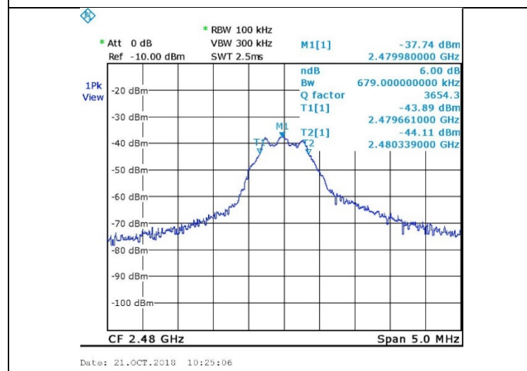
Figure 9. 2480.0 MHz, BLE
