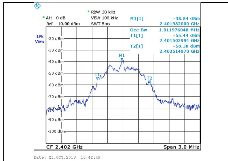
Figure 29. 2402.0 MHz, BLE
