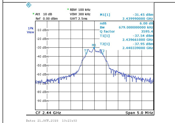
Figure 8. 2440.0 MHz, BLE
