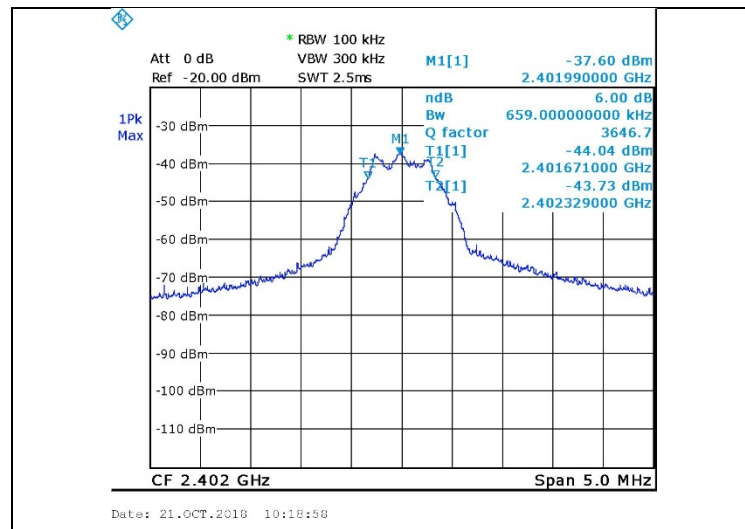
Figure 7. 2402.0 MHz, BLE
