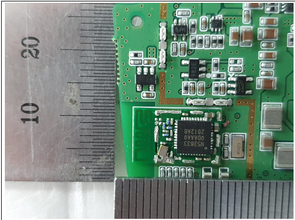
<Main PCB BT_ANT+Module>
