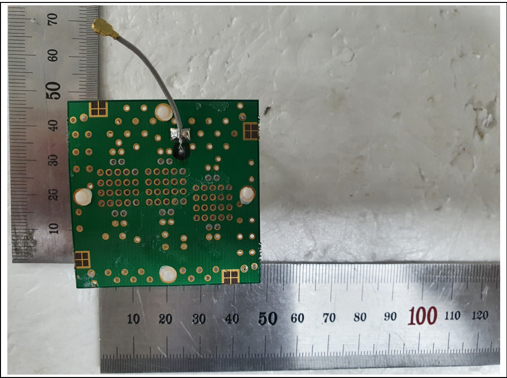
<RFID Antenna>
