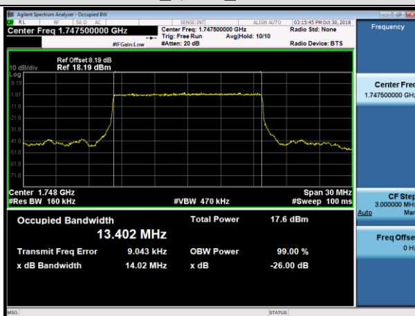
HCH_QPSK_75RB#0
