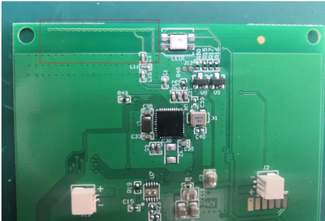
Antenna
