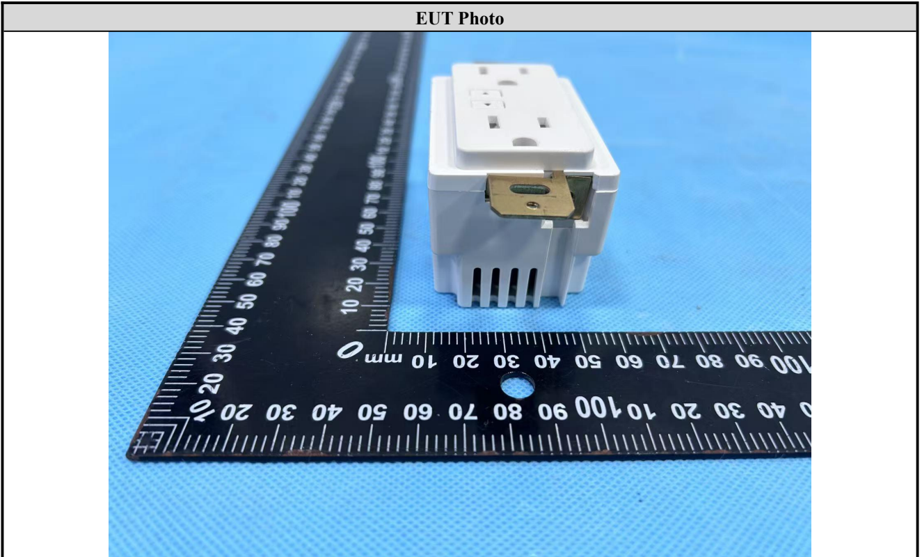
EUT Photo
