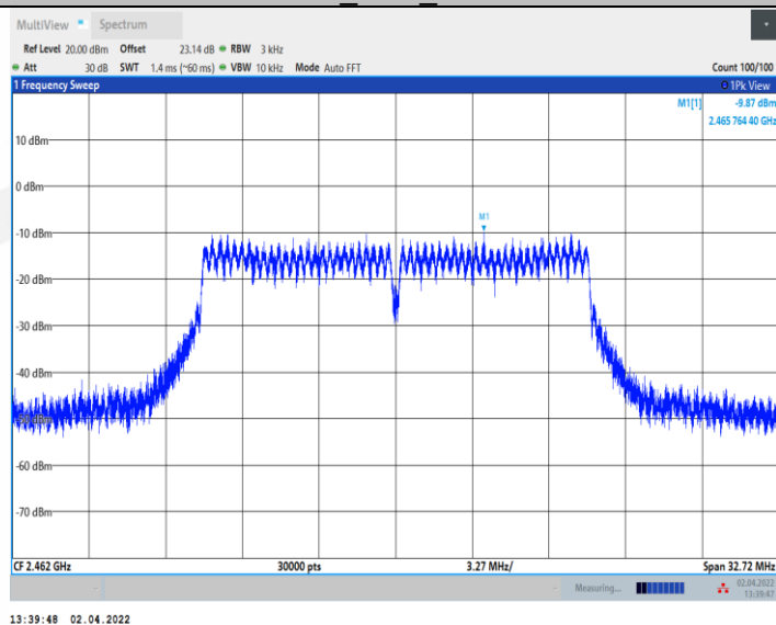
11G_Ant2_2462
