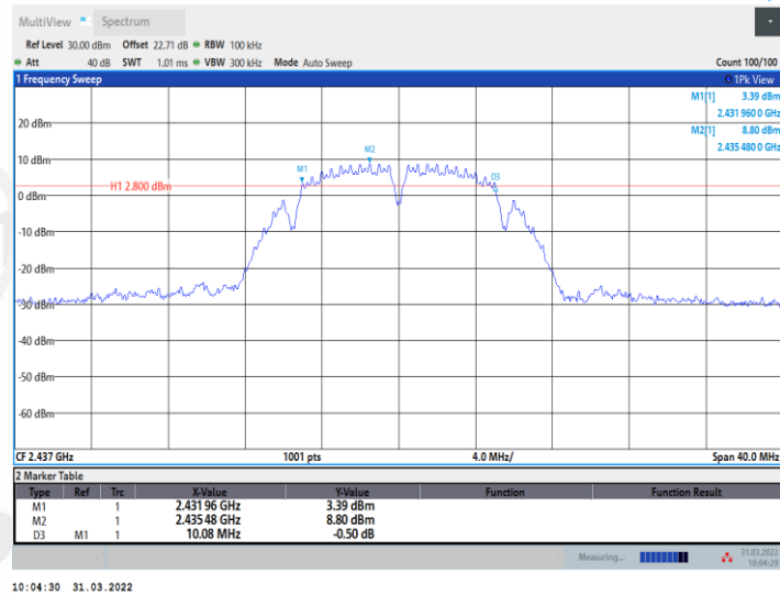
11B_Ant2_2437
