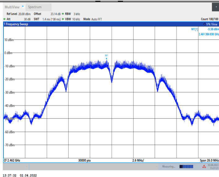
11B_Ant2_2462
