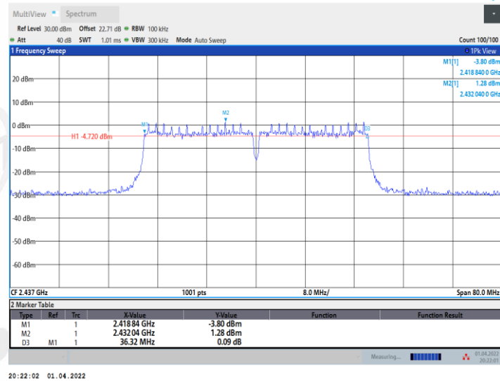
11N40MIMO_Ant2_2437
