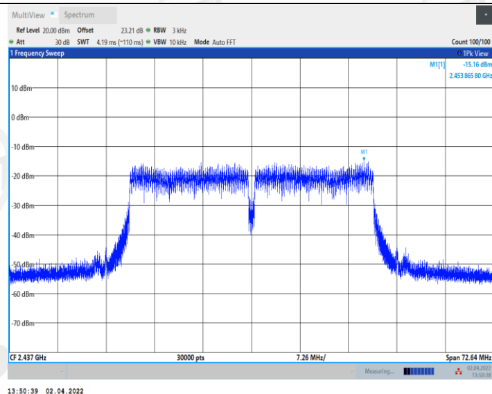
11N40MIMO_Ant2_2437
