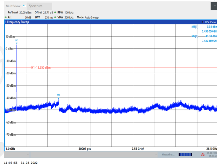
11N20MIMO_Ant2_2437_0~Reference
