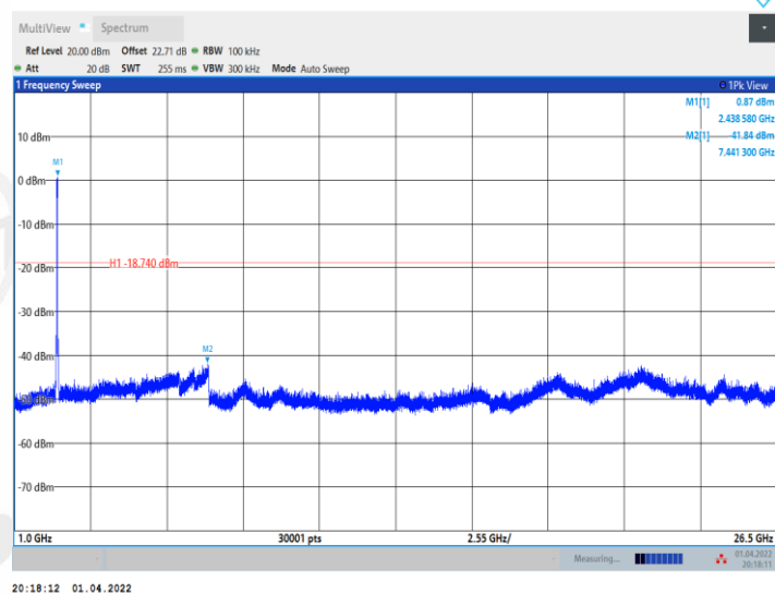
11N40MIMO_Ant2_2422_0~Reference
