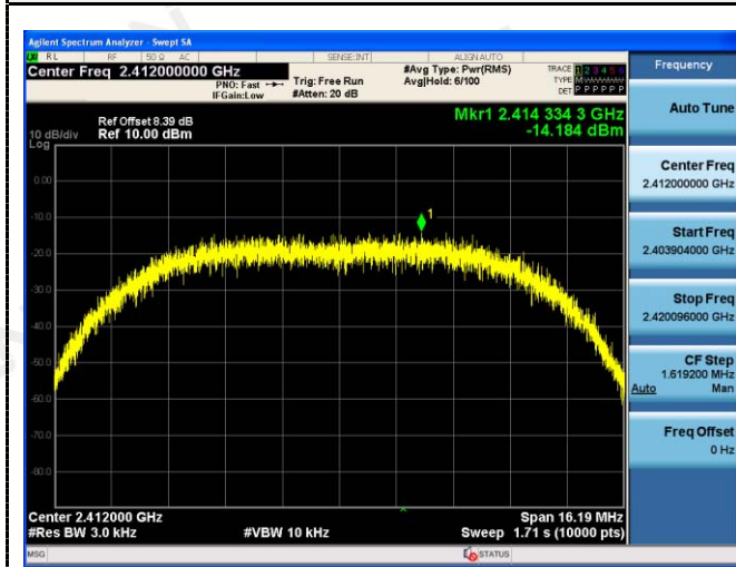
802.11b
