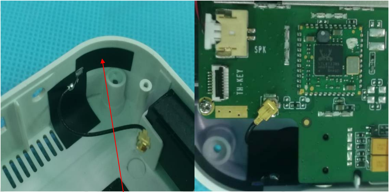
Antenna
