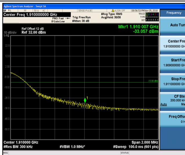
Band2 20MHz QPSK 19100 100RB#0
