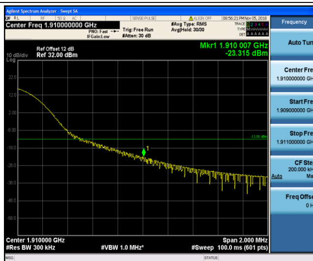
Band2 20MHz QPSK 19100 1RB#99
