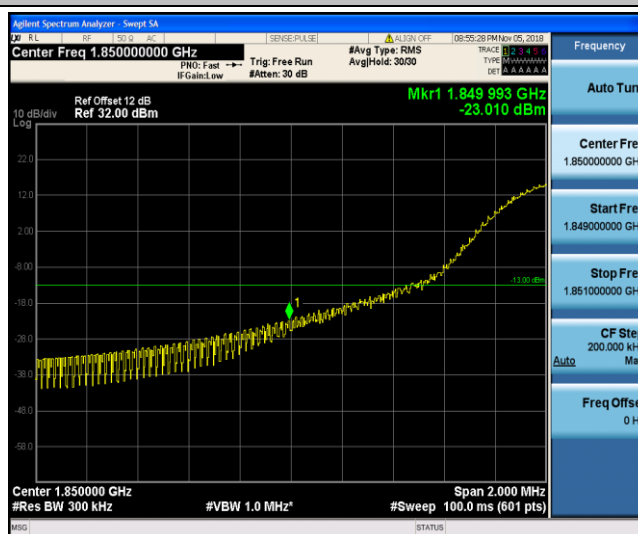
Band2 20MHz 16QAM 18700 1RB#0
