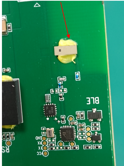
BLE ANT
