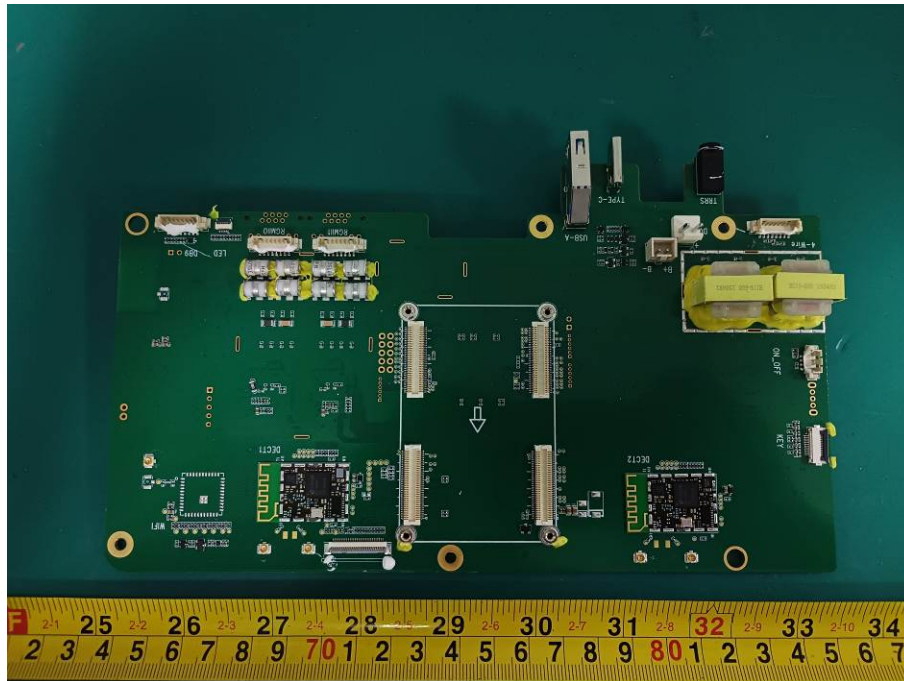
DECT Module 1
