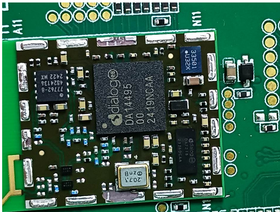
DECT Module 1
