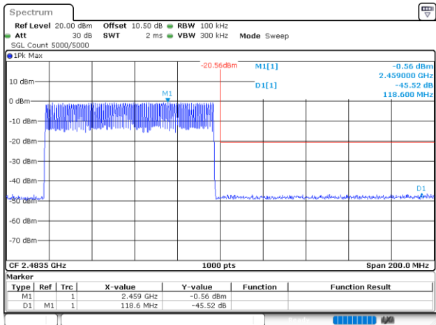
GFSK_Hopping_Upper
