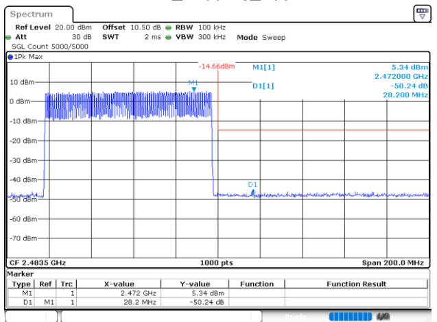
GFSK_Hopping_Upper
