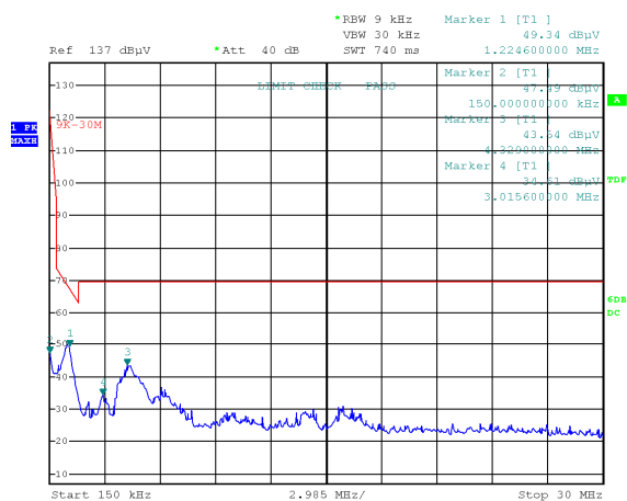
150 kHz -30 MHz
