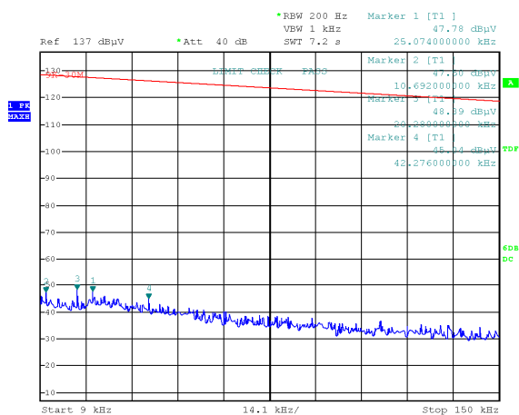
9 kHz-150kHz
