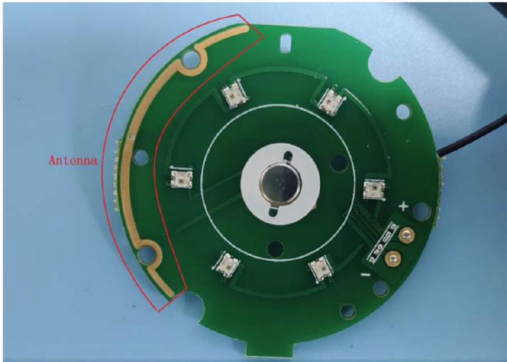
Antenna
