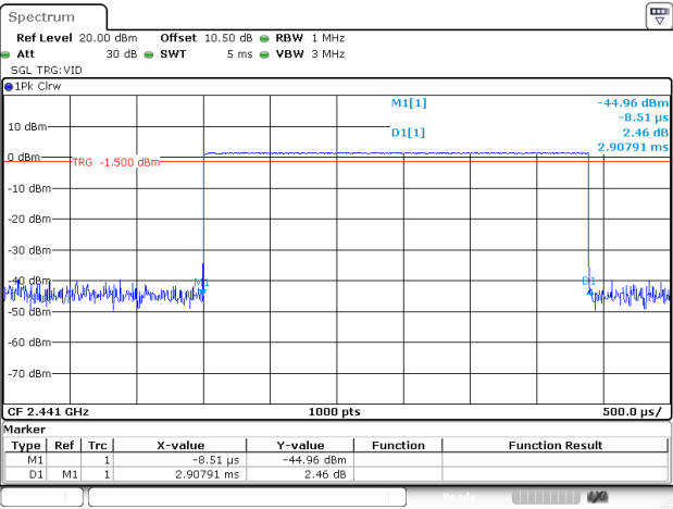
DH5_Hopping
