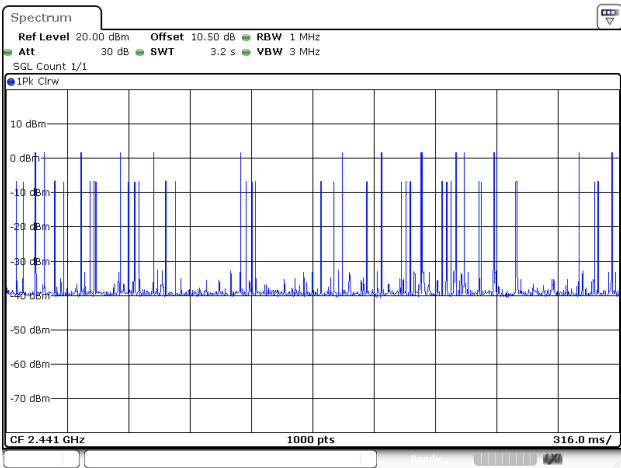
DH3_Hopping
