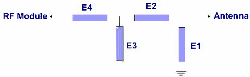
315/433 匹配电路
