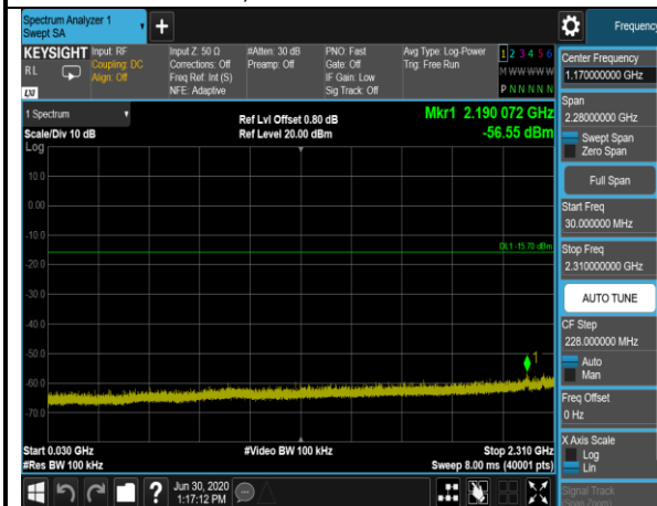
802.11n(HT20),2412MHz,Ant1,Plot 3,30MHz~2310MHz
