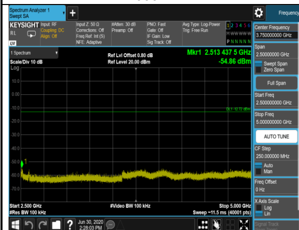
802.11b,2437MHz,Ant1,Plot 4,2500MHz~5000MHz
