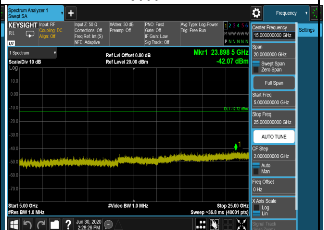
802.11b,2437MHz,Ant1,Plot 5,5000MHz~25000MHz
