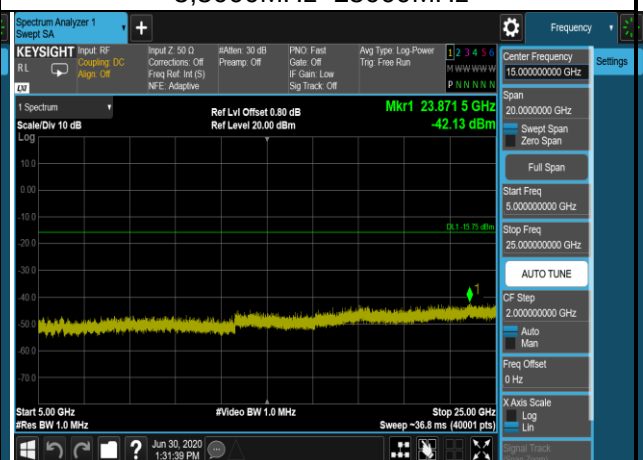
802.11n(HT20),2437MHz,Ant1,Plot 5,5000MHz~25000MHz
