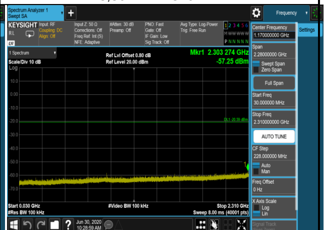
802.11n(HT40),2452MHz,Ant1,Plot 3,30MHz~2310MHz
