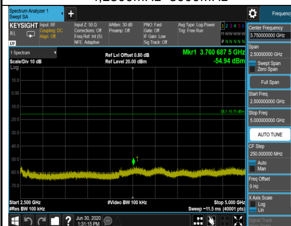
802.11n(HT20),2437MHz,Ant1,Plot 4,2500MHz~5000MHz
