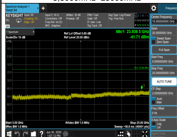
802.11n(HT20),2462MHz,Ant1,Plot 5,5000MHz~25000MHz
